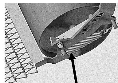
Ressorts tension Décrotoir
